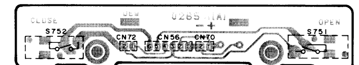
Q SWITCH P.C.B. (REP0421A)
