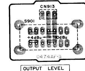
K OUTPUT LEVEL P.C.B. (RFKBV3900EBA)
