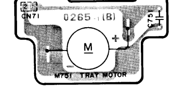
P TRAY MOTOR P.C.B. (REP0421A)
