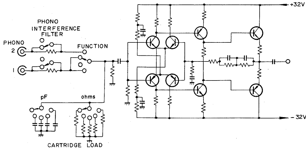
Fig. 5-1 EQ Amplifier
