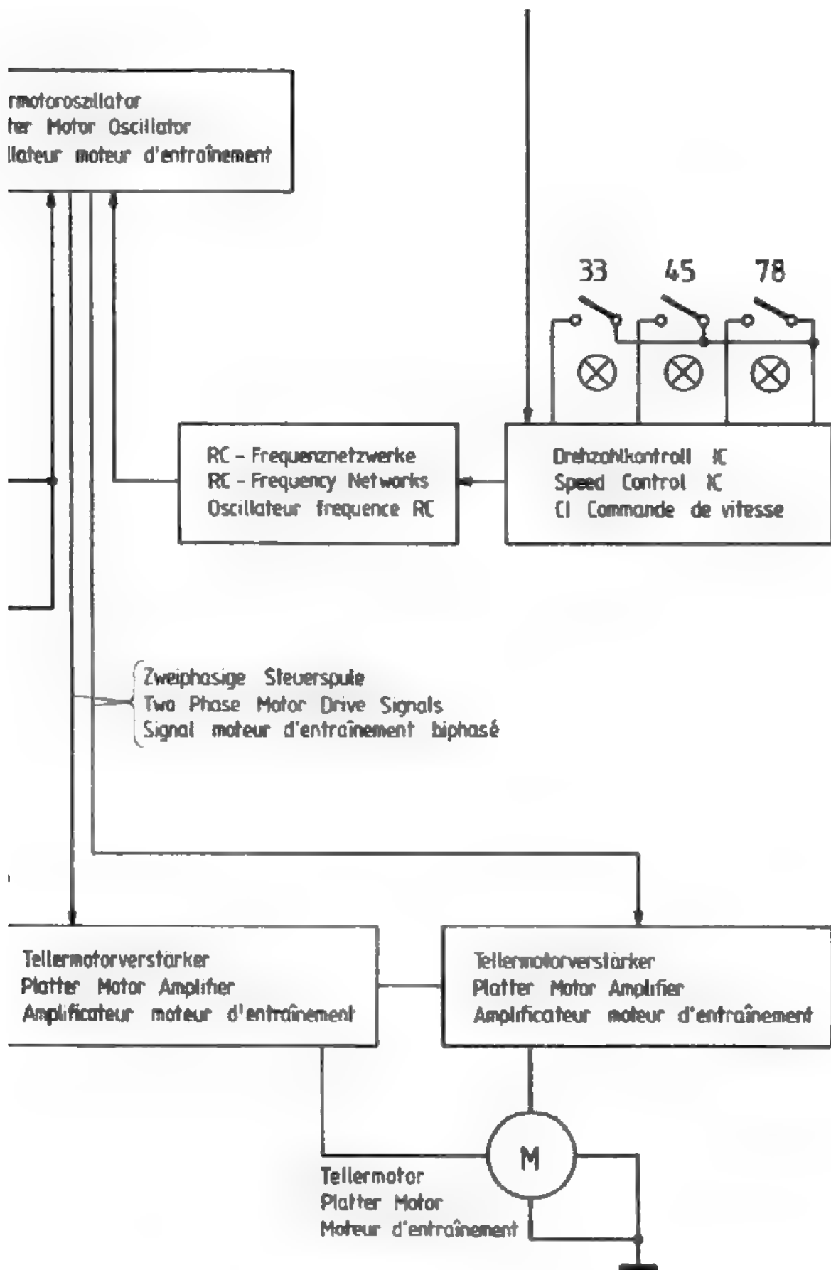
Blockschaltbild Block Diagram
